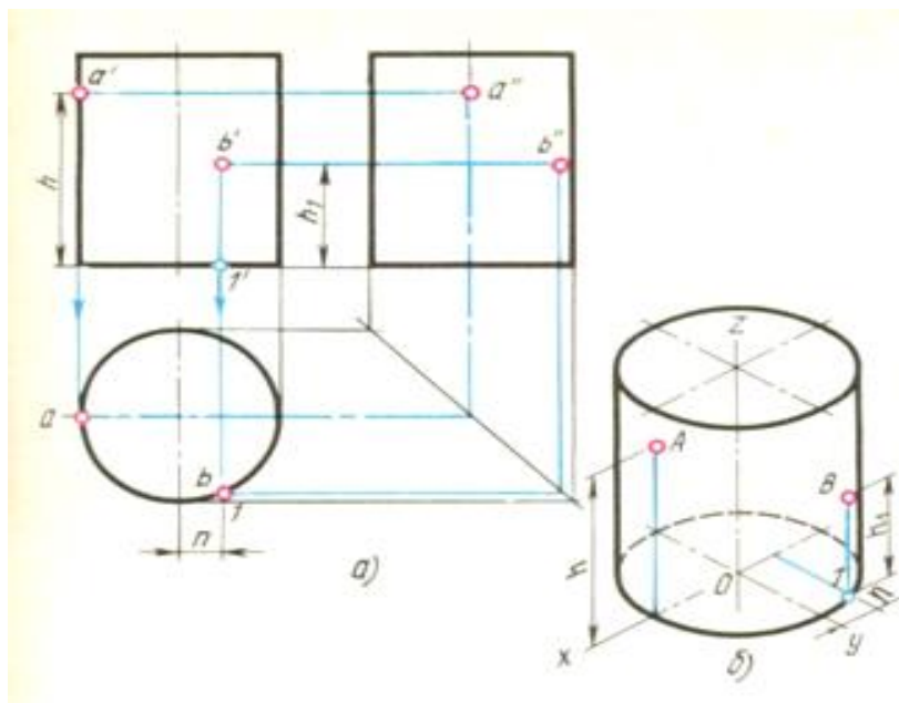
Рисунок 6 – Комплексный чертёж цилиндра и его изометрическая проекция
