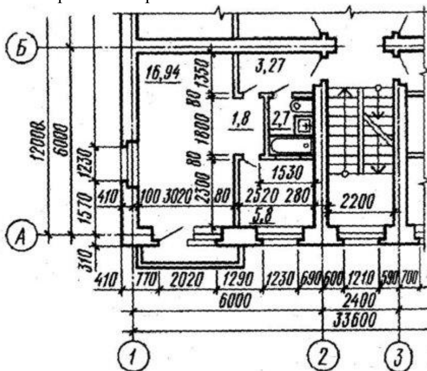
Рисунок 43 - Изображение на плане сантехнического оборудования и простановка размеров
