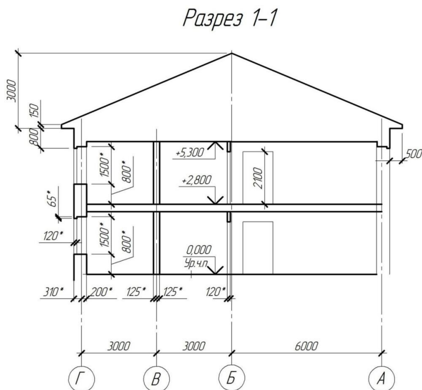
Рисунок 45 – Пример оформления разреза здания
