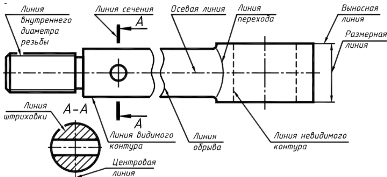
Рисунок 1 – Деталь
