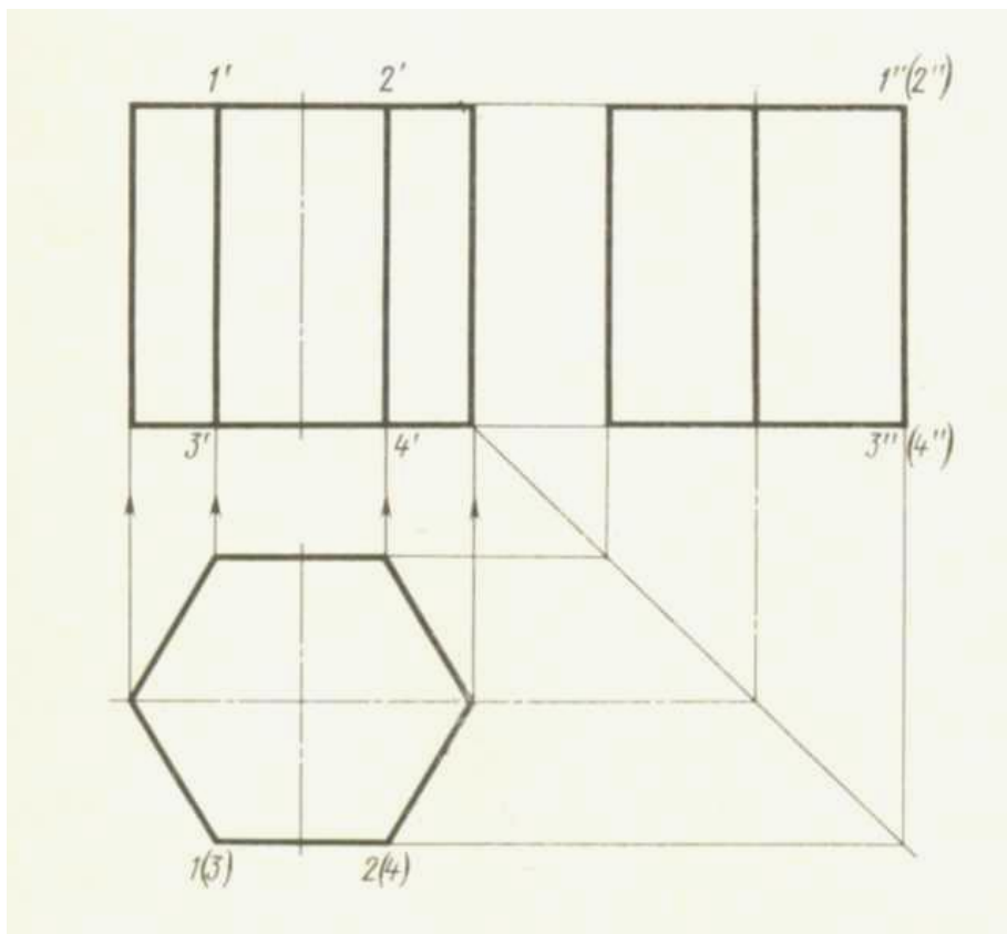
Рисунок 3 – Комплексный чертеж призмы
