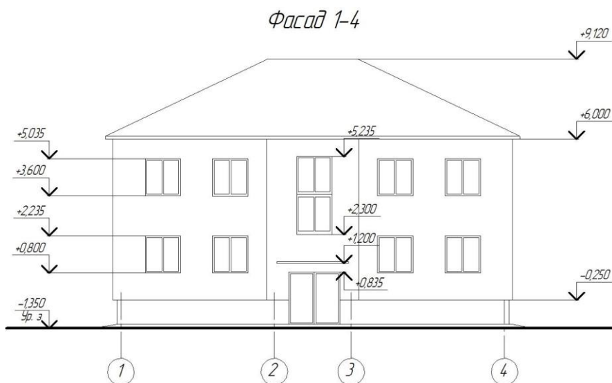
Рисунок 48 - Пример оформления фасада здания
