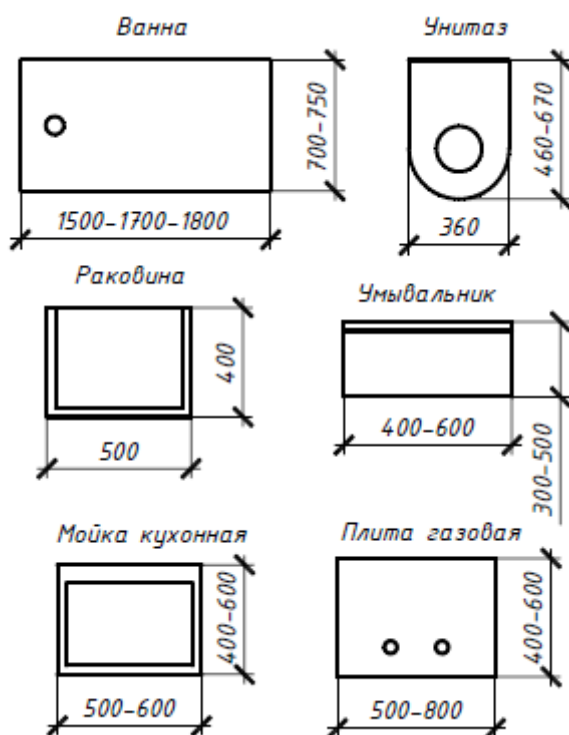
Рис. 39 - Обозначения санитарно-технического оборудования.
