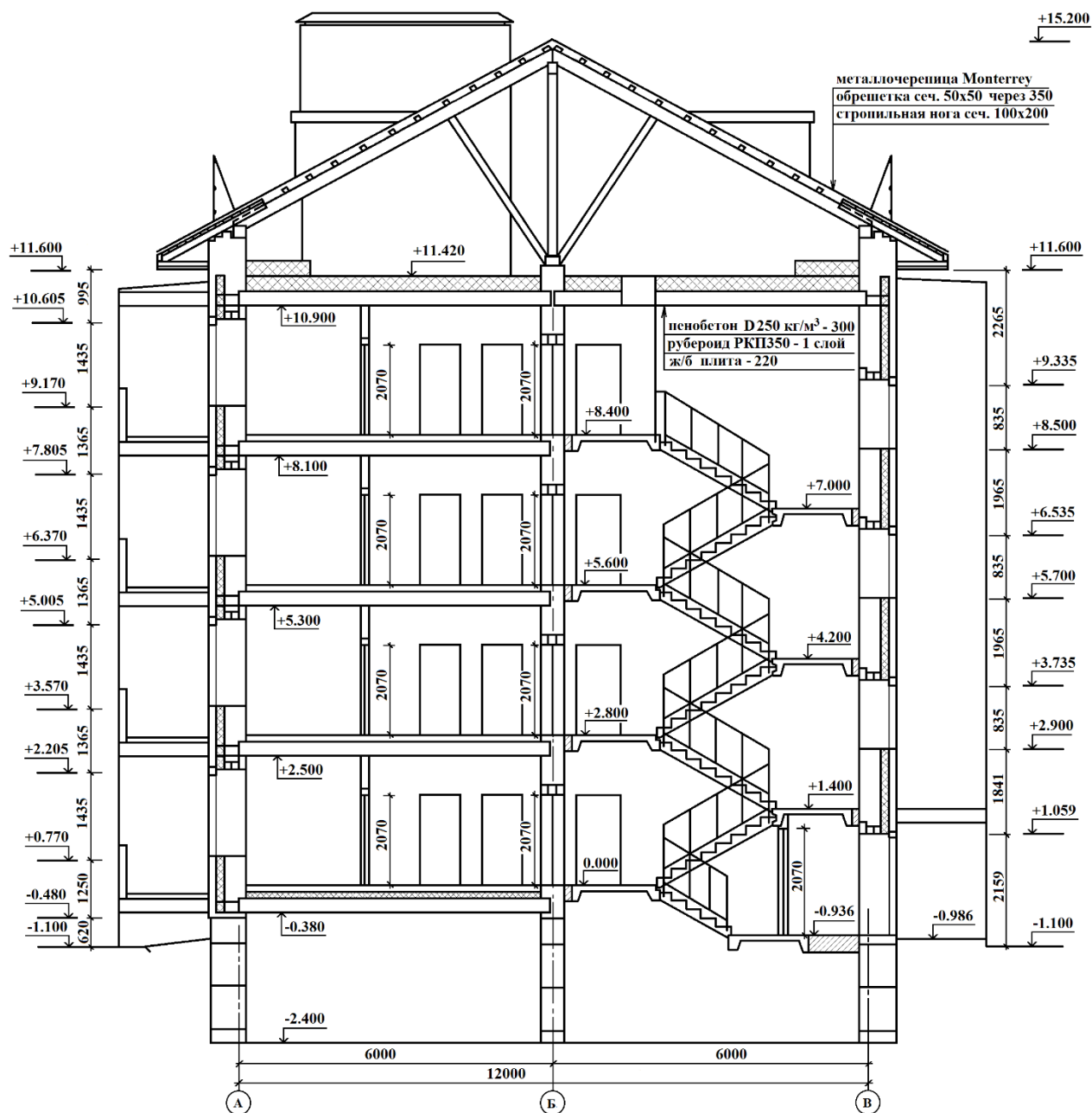
Рисунок 47 –Пример оформления разреза здания
