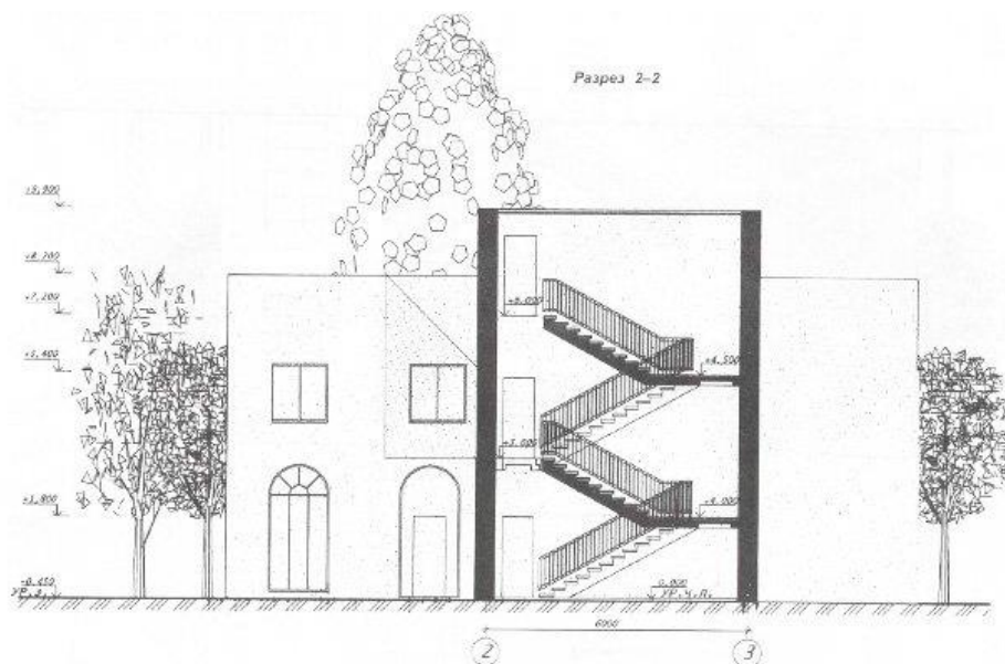
Рисунок 46 – Пример оформления разреза здания
