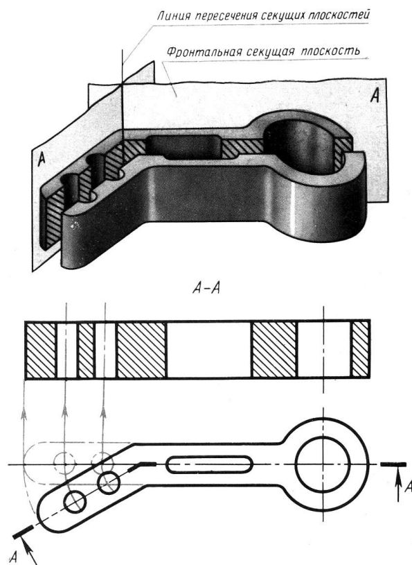
Рисунок 30 – Образование сложного ломаного разреза
