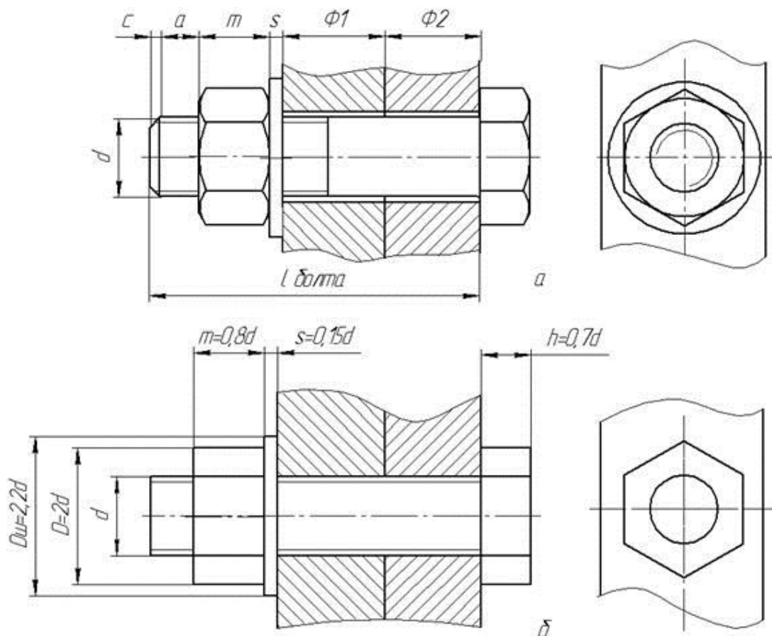
Рисунок 31 – Действительное (а) и упрощенное (б) изображение болтового соединения
