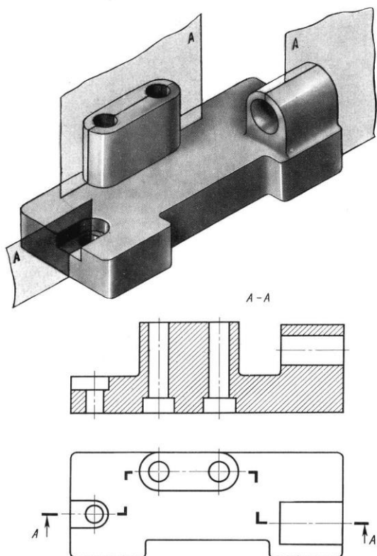
Рисунок 29 – Образование сложного ступенчатого разреза
