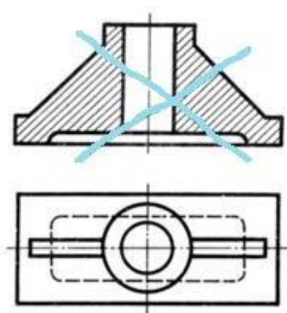
Рисунок 16 - Неправильное построение разреза вдоль тонкого ребра.
