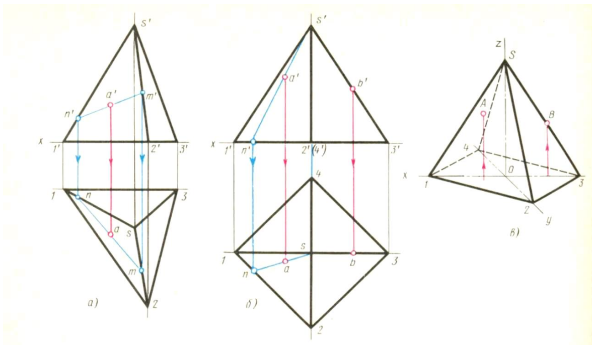
Рисунок 4 - Комплексный чертеж пирамиды
