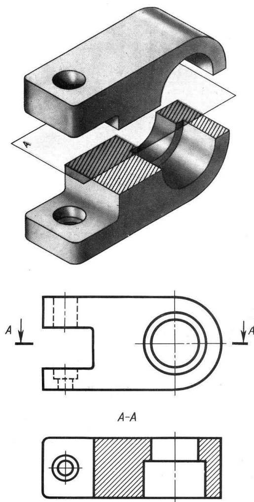
Рисунок 12 - Образование простого профильного разреза
