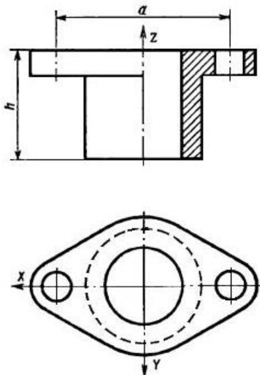
Рисунок 22. Чертеж крышки сальника.
