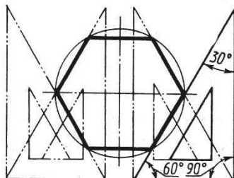
Разделить окружность на 6 и 8 равных частей
