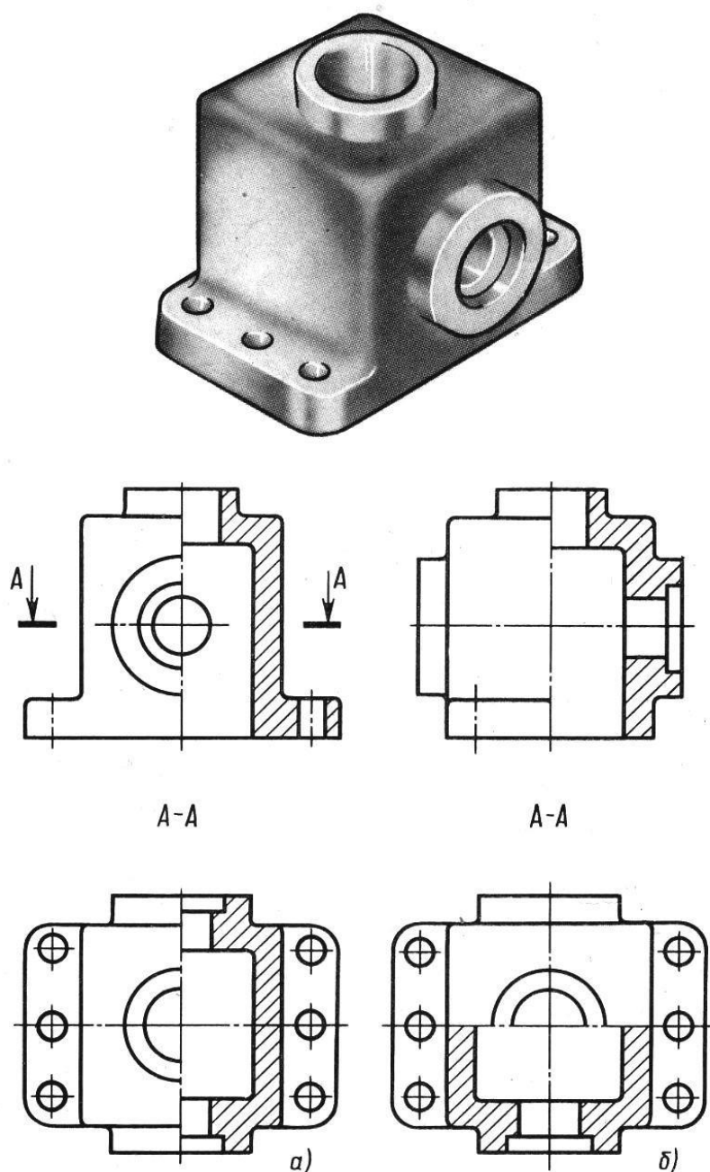
Рисунок 13 - Совмещение вида с разрезом
