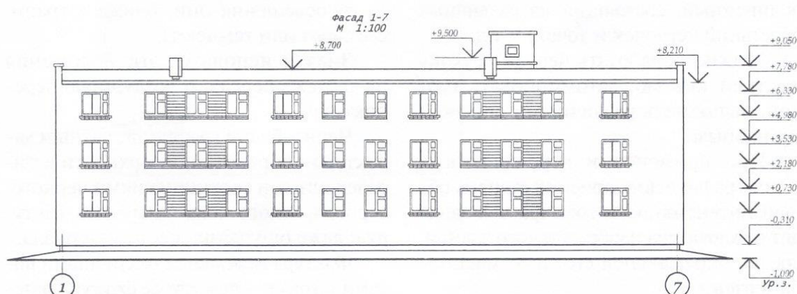
Рисунок 49 - Пример оформления фасада здания.
