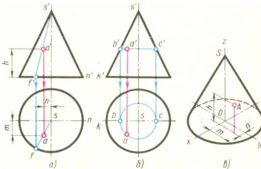
Рисунок 8 – Комплексный чертеж конуса и его изометрическая проекция
