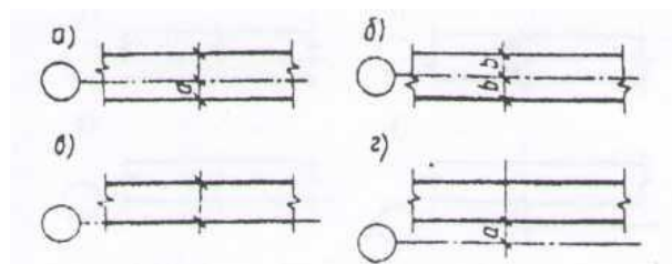
Рисунок 44 –Виды привязок:
