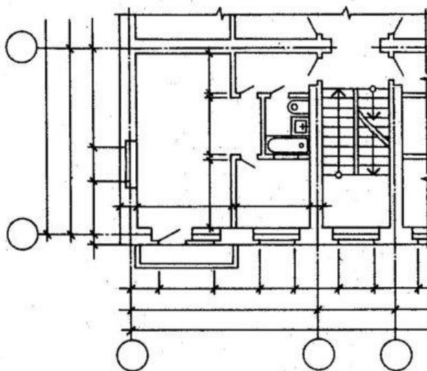
Рисунок 42 - Нанесение оконных и дверных проемов, лестниц и площадок
