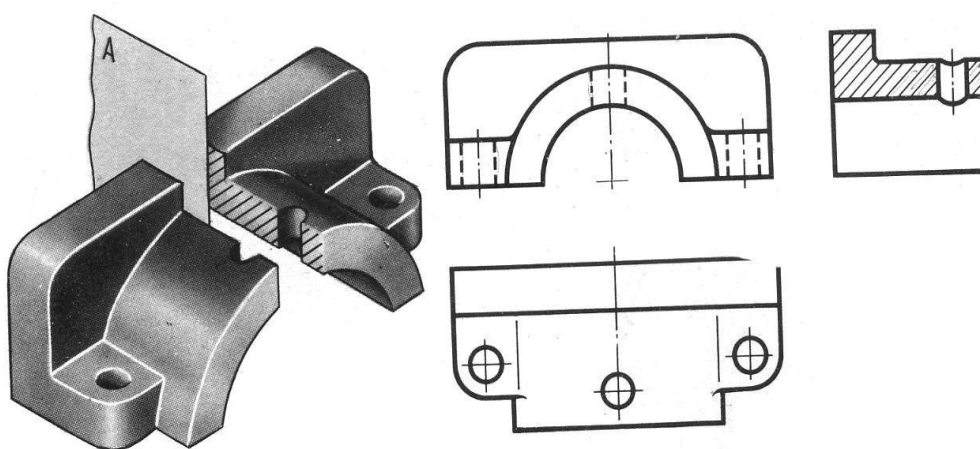
Рисунок 11 - Образование простого профильного разреза
