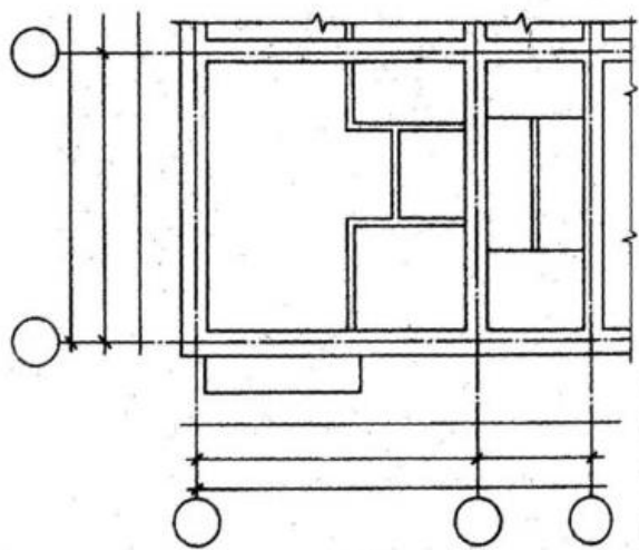
Рисунок 41 - Нанесение на плане стен здания
