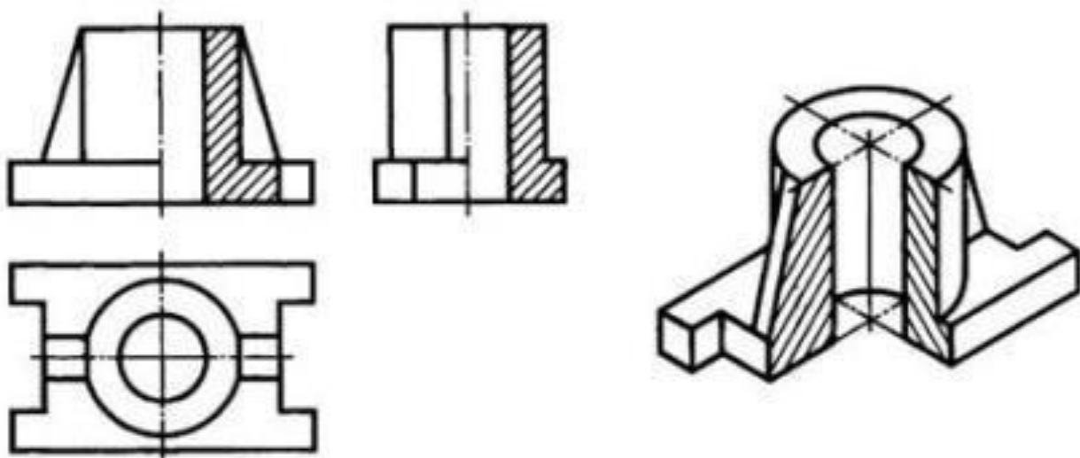
Рисунок 17 – Чертеж детали
